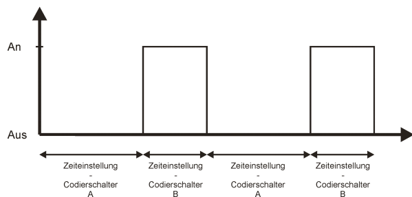
Signalfolge - Codierschalter- / Zeitzuordnung
