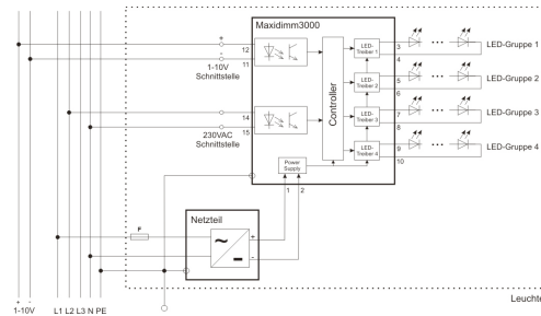
Blockschema und Verkabelung der Leitungen
