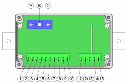
Anschlussbelegung und Codierschalterzuordnung
